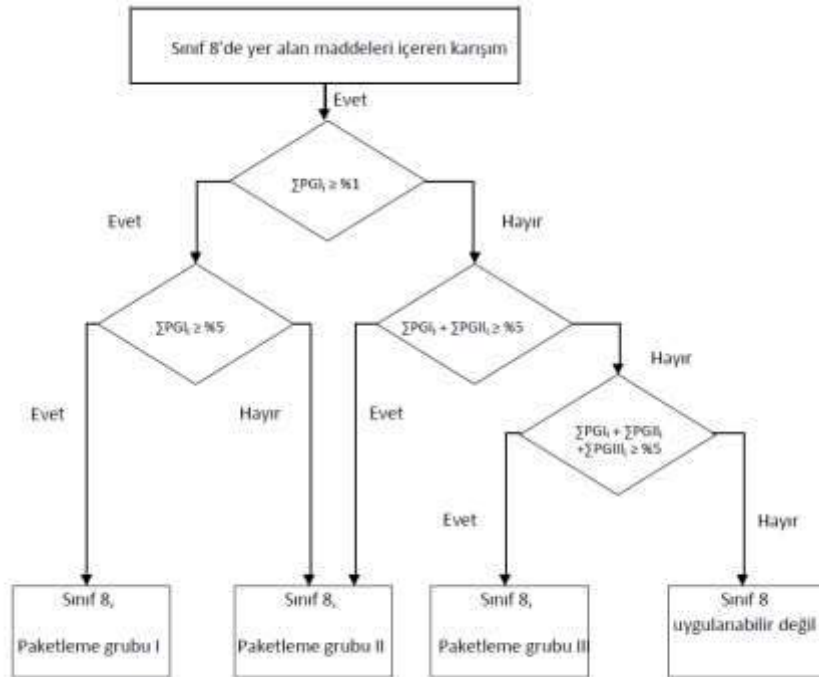
Şekil 2.2.8.1.6.3: Hesaplama yöntemi
