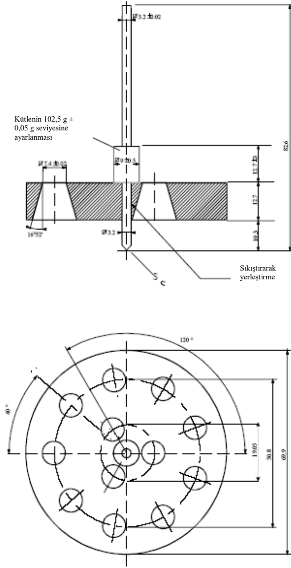
Şekil 1 - Penetrometre
